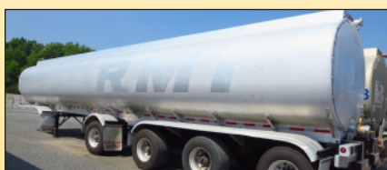
Citerne REMTEC 2008 , 57,000 litres, aluminium, convertie en 1 compt. avec plaques anti vagues, choix de valve de sortie arrière, idéal pour le tsp. de produits non placardés, inclus inspection SAAQ et teste d'étanchéité
