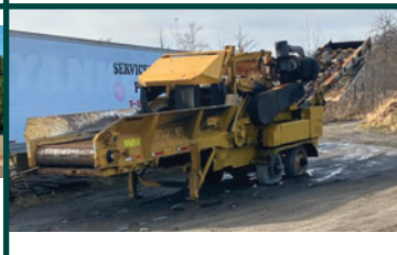
Convoyeur incendié et filages HG4000 , (chipper à bois) 2016, 3,500 heures $ 30 000 Tél.: 418-872-3660
