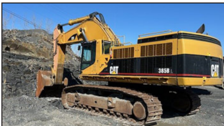
Unité : 5102 Excavatrice hydraulique CAT 385B 2002 , 25,950 heures, moteur rebâti, pompe rebâti Prix: 135 000 $
