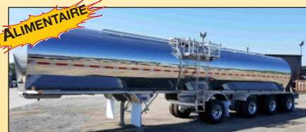
Citerne TREMCAR , 38,000 litres alimentaire, neuve, tuyauterie pour lavage intérieur, coffre arrière, rampe de sécurité sur le haut
