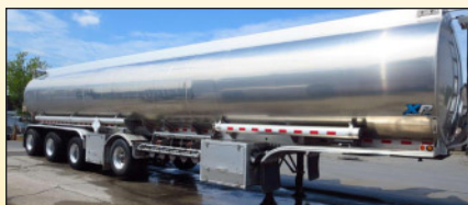
Citerne REMTEC 2017 , 57,000 litres, 6 compt., pour produits pétroliers, 2 coffres, 5 tubes pour boyaux, inclus inspection SAAQ et B-620
