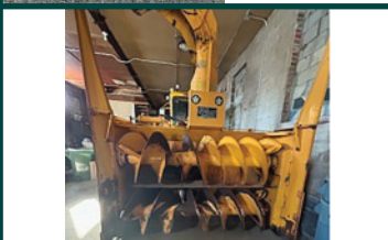
Souffleuse VOHL , bonne condition, pneus neufs, moteur Ford avant et moteur GM arrière $ 9 500 Tél.: 514-977-3450 / 450-427-3450
