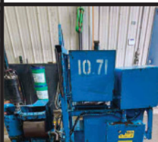
Processeur à bois chauffage , K-415 diesel mobile P.S.D. Tél.: 819-372-6392
