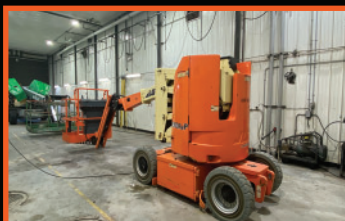
JLG E450AJ 2016, 2x4, électrique
