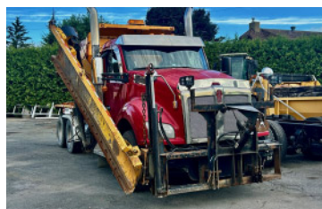
KENWORTH T880 2017 , Paccar 485 hp, Ultrashift 18, 16/46 "Full Lock", équipement à neige complet Tenco, Dickey John
