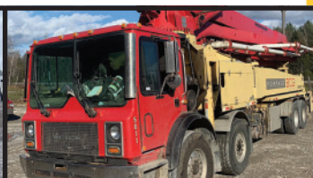
Pompe à béton Schwing et Putzmeister 31M, 32M, 39M et 42M, sur Mack MR 2007, très bonne condition
