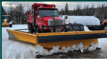
FREIGHTLINER M2-112V 2011, moteur DD 13-450 hp, transm. Eaton-Fuller RTO- 16908LL 18 vitesses, 221,626 km Prix de base suggéré $ 50 000 Tél.: 819-326-2674 Poste: 3400
