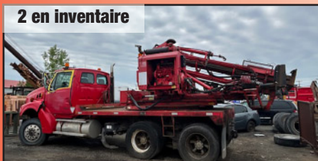
Planteur à pieu sur camion, équipé de mot. stationnaire 4 cyl. JD, peu vendre séparément
