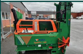
Processeur à bois chauffage, K-415 de Posch
