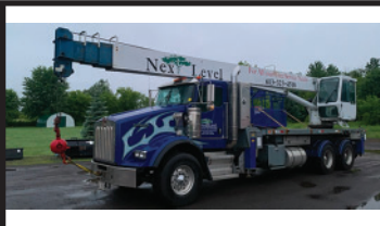
2010 MANITEX 30112 monté sur Kenworth T-880, Cummins ISM, 380,919 km P.S.D. Tél.: 450-467-2642 Poste: 1209
