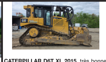
CATERPILLAR D6T XL 2015 , très bonne condition malgré son nombre d'heures (16 521), mot. Cat C9.3 ACERT 228 hp, cabine fermée avec A/C et chauffage, etc. $ 93 000 Tél.: 450-471-1111
