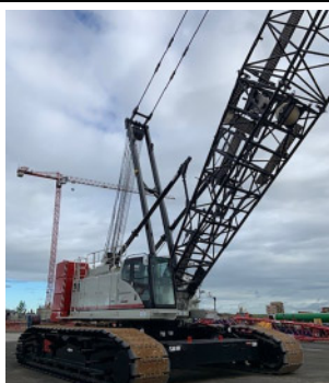
2025 LINK-BELT 248HSL , flèche 205', fléchette 60' et tête auxiliaire, huile bio, LMI avec coupe hydraulique
