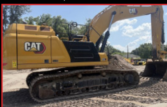
CATERPILLAR 352 2023 , 4,000 heures, système 2D, filage GPS, balance intégrée
